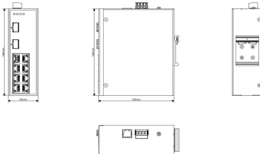
交换机尺寸图
