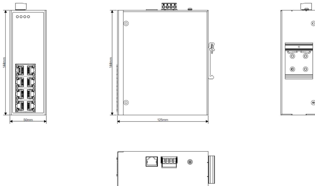
交换机尺寸图
